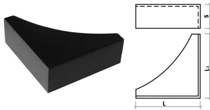
PROTEGGIANGOLO 70X70X26
