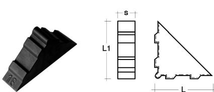
PROTEGGIANGOLO 55X55X16
