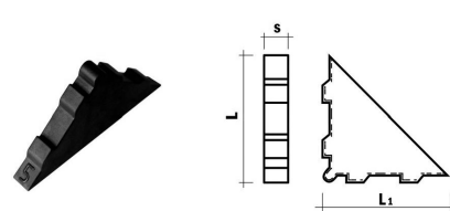
PROTEGGIANGOLO 55X55X5
