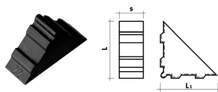
PROTEGGIANGOLO 55X55X22
