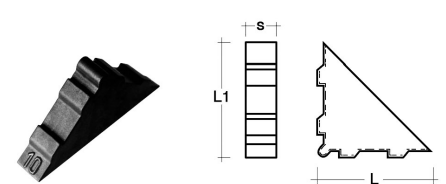
PROTEGGIANGOLO 55X55X10
